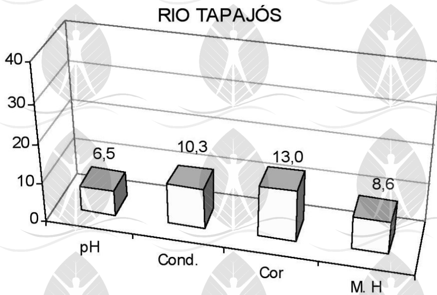
Figura-92. Mostra os valores de pH, condutividade elétrica ( \mu\text{S}/\text{cm} ), cor ( \text{mg}/\text{Pt}/\text{L} ) e material húmico (M.H) no rio Tapajós (SANTOS e RIBEIRO, 1988).
