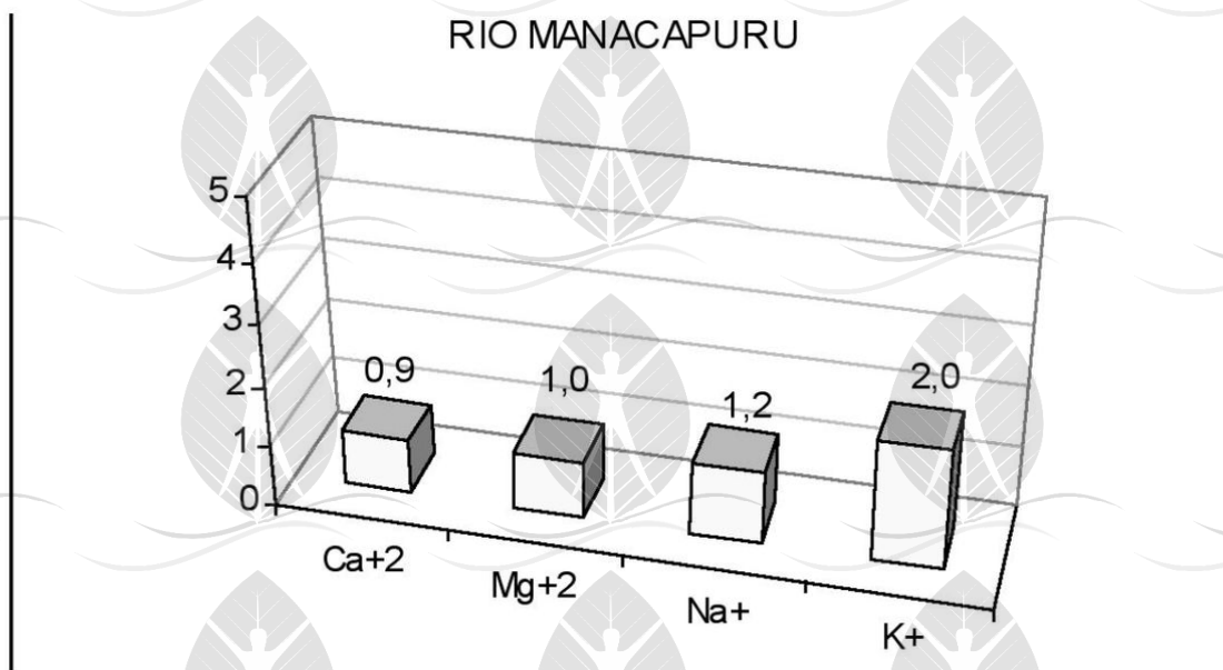
Figura-54. Mostra os valores de cálcio (Ca +2 ), magnésio (Mg +2 ), sódio (N + ) e potássio (K + ) no rio Manacapuru (SANTOS e RIBEIRO, 1988).
