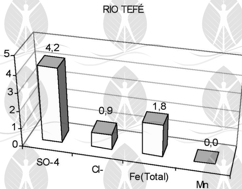
Figura-35. Mostra os valores de sulfato (SO 4 - ), cloreto (Cl - ), ferro total (Fe) e manganês (Mn) no rio Tefé (SANTOS e RIBEIRO, 1988).
