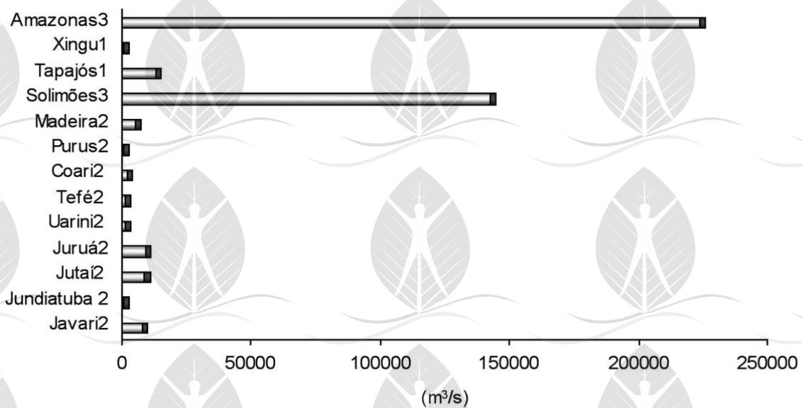
Figura-110: Mostra a vazão de afluentes da margem direita e do Amazonas no período de cheia (1 - HIBAM Campanha Solimões-Amazonas, 1997; 2 - HIBAM Campanha Solimões-Amazonas, 2002 e 3 - HIBAM Campanha Solimões-Amazonas, 2003).
