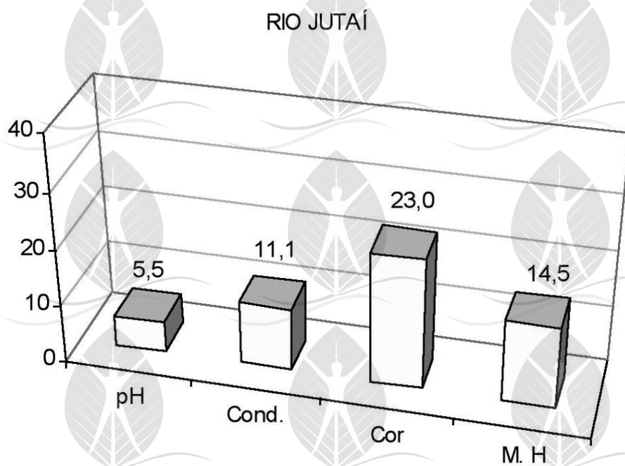
Figura-18. Mostra os valores de pH, condutividade elétrica ( \mu\text{S}/\text{cm} ), cor ( \text{mg}/\text{Pt}/\text{L} ) e material húmico (M.H) no rio Jutai (SANTOS e RIBEIRO, 1988).
