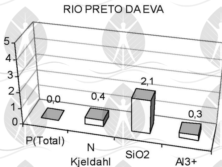
Figura-66. Mostra os valores de fósforo total (Pt), nitrogênio (Nk), silicato (SiO 2 ) e alumínio (Al+3) no rio Preto da Eva (SANTOS e RIBEIRO, 1988).
