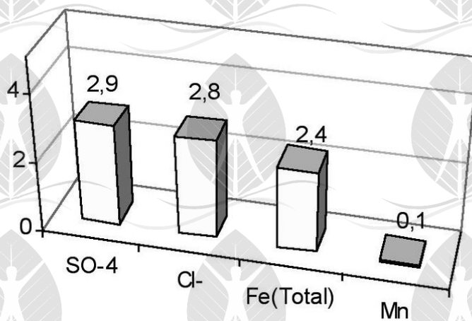
Figura-30. Mostra os valores de sulfato (SO 4 - ), cloreto (Cl - ), ferro total (Fe) e manganês (Mn) no rio Juruá (SANTOS e RIBEIRO, 1988).
