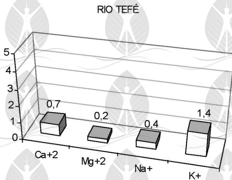
Figura-34. Mostra os valores de cálcio (Ca+2), magnésio (Mg+2), sódio (N+) e potássio (K+) no rio Tefé (SANTOS e RIBEIRO, 1988).
