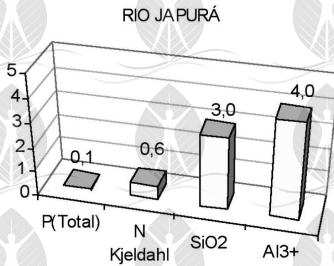
Figura-26. Mostra os valores de fósforo total (Pt), nitrogênio (Nk), silicato (SiO 2 ) e alumínio (Al 3+ ) no rio Japurá (SANTOS e RIBEIRO, 1988).
