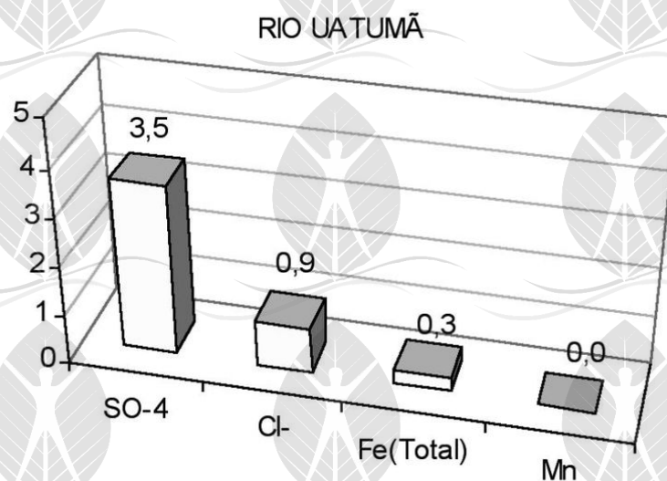
Figura-79. Mostra os valores de sulfato (SO 4 - ), cloreto (Cl - ), ferro total (Fe) e manganês (Mn) no rio Uatumã (SANTOS e RIBEIRO, 1988).
