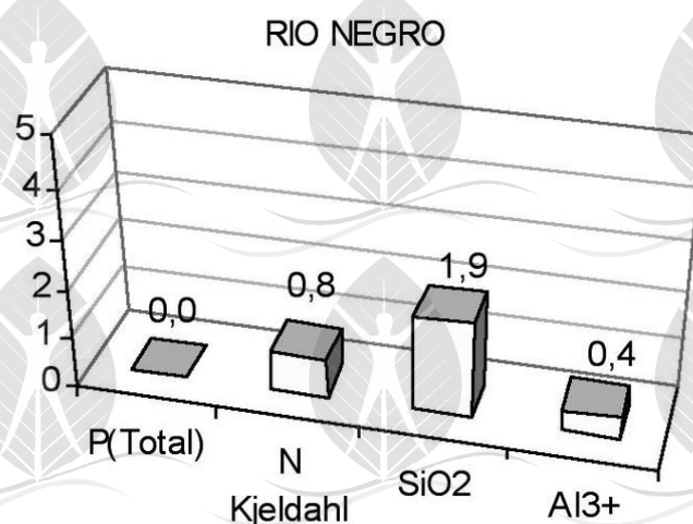
Figura-61. Mostra os valores de fósforo total (Pt), nitrogênio (Nk), silicato (SiO 2 ) e alumínio (Al+3) no rio Negro (SANTOS e RIBEIRO, 1988).
