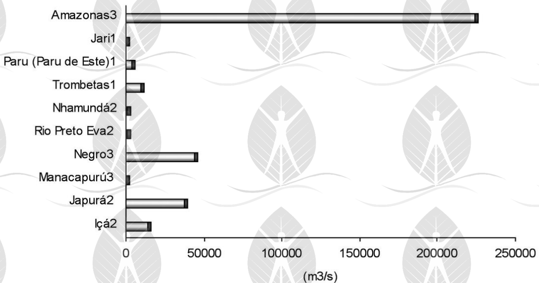
Figura-111. Mostra a vazão de afluentes da margem esquerda e do Amazonas no período de cheia (1 = HIBAM Campanha Solimões-Amazonas, 1997; 2 = HIBAM Campanha Solimões-Amazonas, 2002 e 3 = HIBAM Campanha Solimões-Amazonas, 2003).
