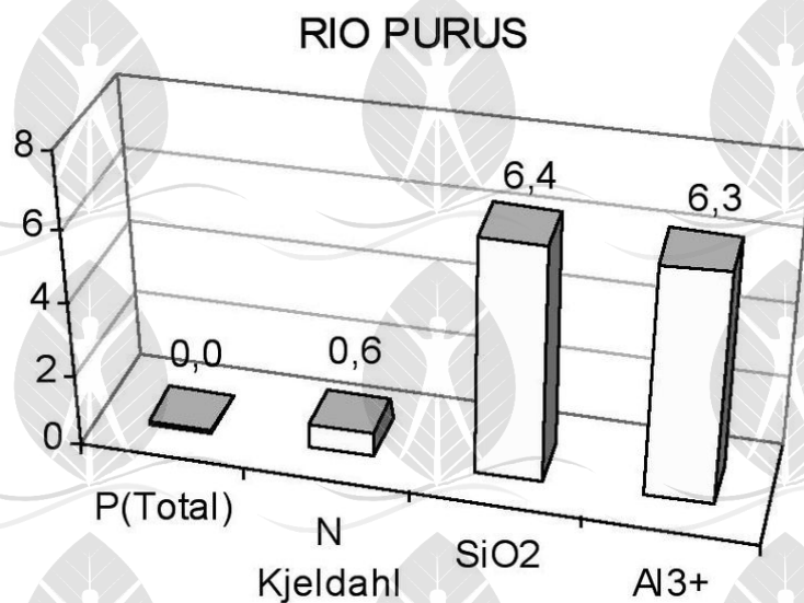
Figura-46. Mostra os valores de fósforo total (Pt), nitrogênio (Nk), silicato (SiO 2 ) e alumínio (Al+3) no rio Purus (SANTOS e RIBEIRO, 1988).
