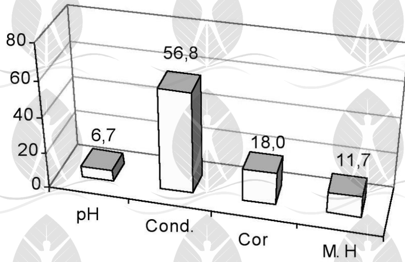
Figura-48. Mostra os valores de pH, condutividade elétrica ( \mu\text{S}/\text{cm} ), cor ( \text{mg}/\text{Pt}/\text{L} ) e material húmico (M.H) no rio Madeira (SANTOS e RIBEIRO, 1988).
