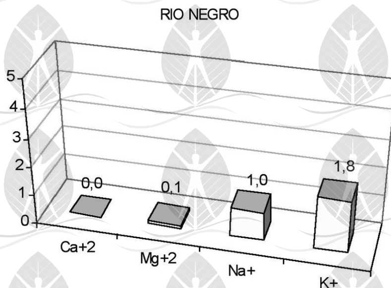
Figura-59. Mostra os valores de cálcio (Ca 2+ ), magnésio (Mg 2+ ), sódio (N + ) e potássio (K + ) no rio Negro (SANTOS e RIBEIRO, 1988).
