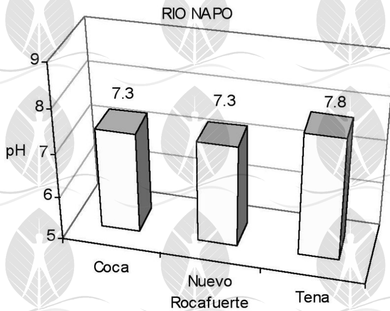
Figura-5. Valores de pH ao longo do rio Napo, em Coca, Nuevo Rocafuerte e Tena (GUYOT et al. 1998).
