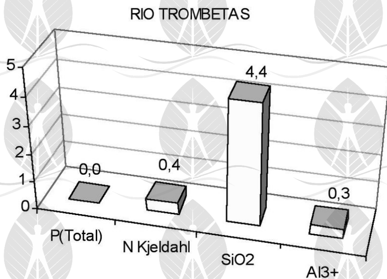
Figura-90. Mostra os valores de fósforo total (Pt), nitrogênio (Nk), silicato (SiO 2 ) e alumínio (Al 3+ ) no rio Trombetas (SANTOS e RIBEIRO, 1988).
