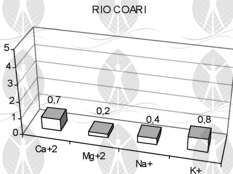
Figura-39. Mostra os valores de cálcio (Ca+2), magnésio (Mg+2), sódio (N+) e potássio (K+) no rio Coari (SANTOS e RIBEIRO, 1988).
