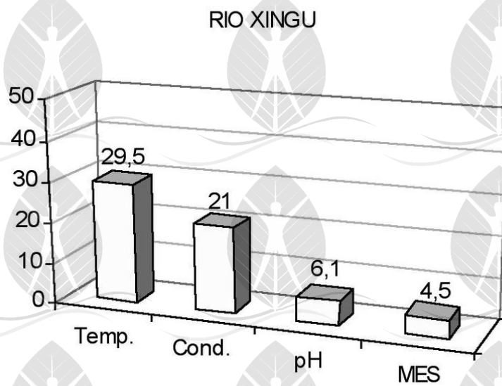
Figura-103. Mostra os valores de temperatura (oC), condutividade ( \mu\text{S}/\text{cm} ), pH e material em suspensão (MES - mg/L) no rio Xingú (HIBAM, 1998).
