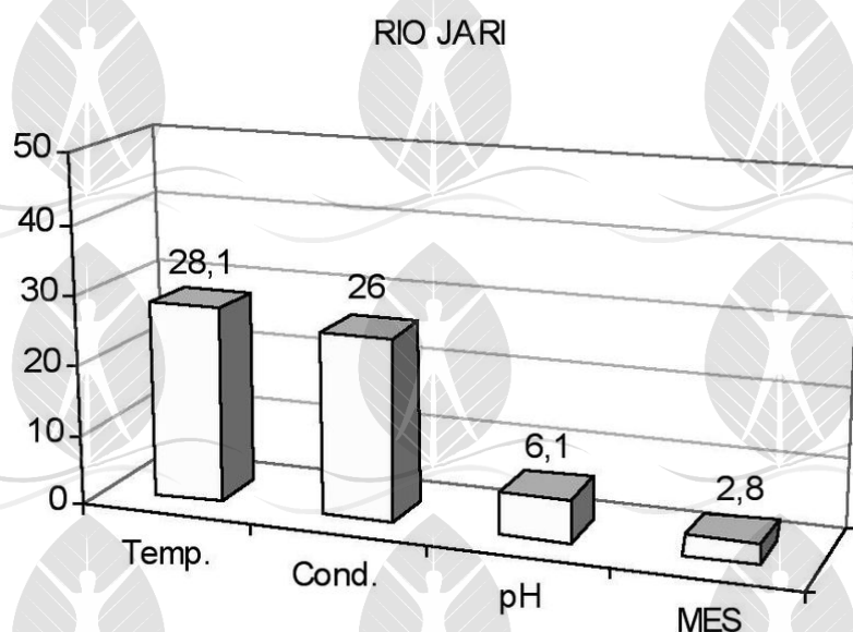
Figura-101. Mostra os valores de temperatura (°C), condutividade ( \mu\text{S}/\text{cm} ), pH e material em suspensão (MES - mg/L) no rio Jari (HIBAM, 1998).
