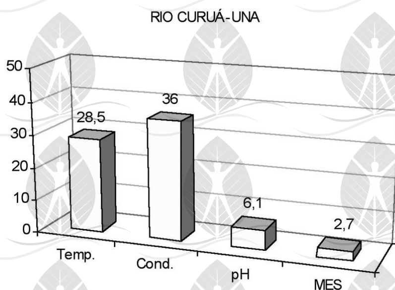
Figur-97. Mostra os valores de temperatura ( ^{\circ}\text{C} ), condutividade ( \mu\text{S}/\text{cm} ), pH e material em suspensão (MES - mg/L) no rio Curuá-Una (HIBAM, 1998).
