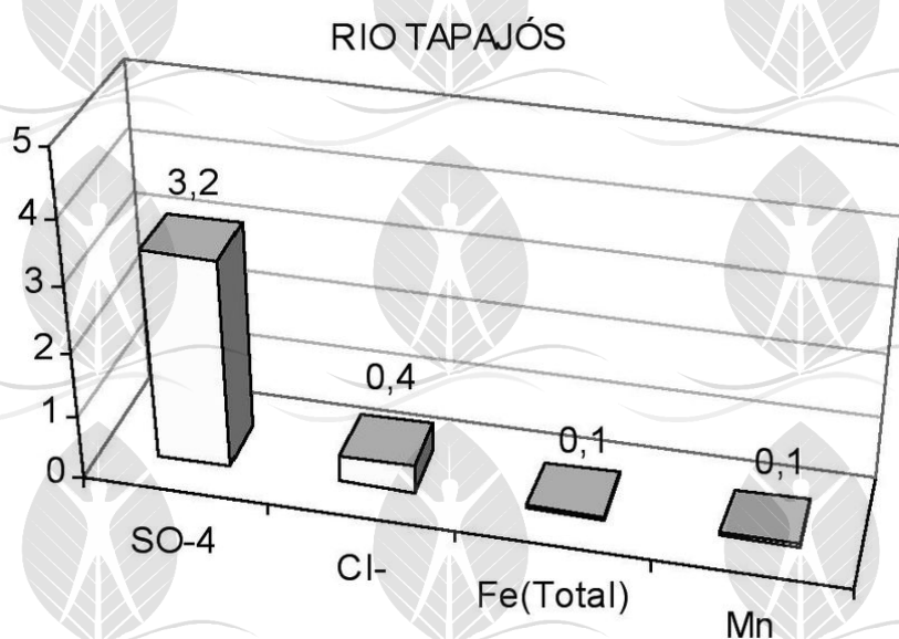
Figura-94. Mostra os valores de sulfato (SO 4 - ), cloreto (Cl - ), ferro total (Fe) e manganês (Mn) no rio Tapajós (SANTOS e RIBEIRO, 1988).
