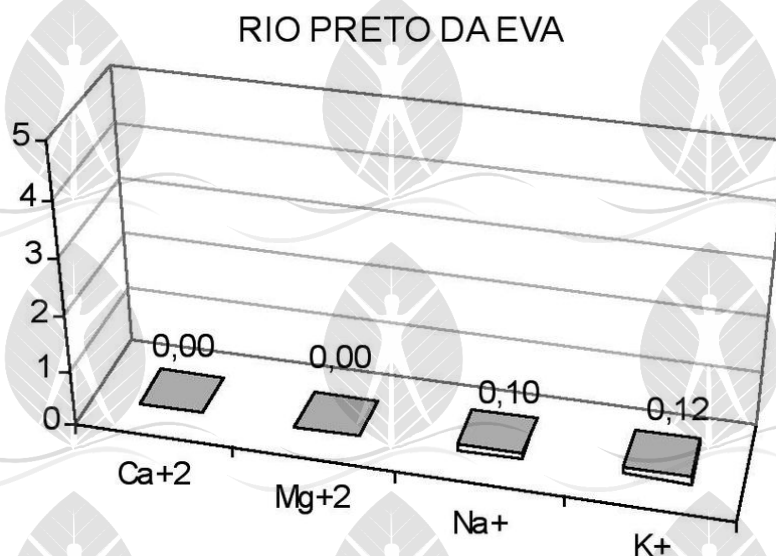
Figura-64. Mostra os valores de cálcio (Ca +2 ), magnésio (Mg +2 ), sódio (N + ) e potássio (K + ) no rio Preto da Eva (SANTOS e RIBEIRO, 1988). Suas águas também apresentaram baixa concentração de ânions, cujo valor médio foi de 0,87 mg/L, com predominância de sulfato (Figura 65).
