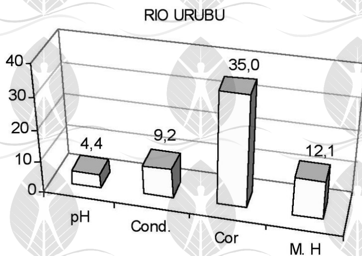
Figura-68. Mostra os valores de pH, condutividade elétrica ( \mu\text{S}/\text{cm} ), cor ( \text{mg}/\text{Pt}/\text{L} ) e material húmico (M.H) no rio Urubu (SANTOS e RIBEIRO, 1988).
