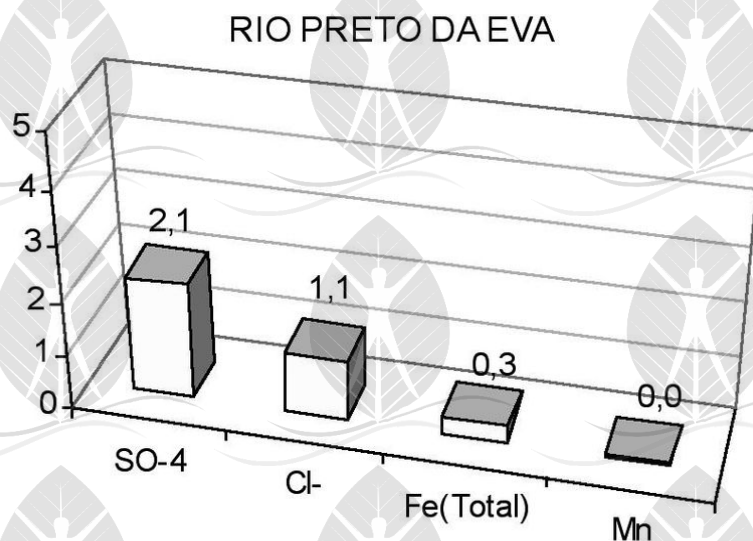
Figura-65. Mostra os valores de sulfato (SO 4 - ), cloreto (Cl - ), ferro total (Fe) e manganês (Mn) no rio Preto da Eva (SANTOS e RIBEIRO, 1988).
